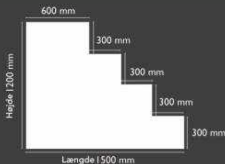
Tegningen viser gav- og helgavlstrappe med fire trappetrin set lige fra siden
